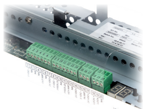
Plug & Play csatlakozók
