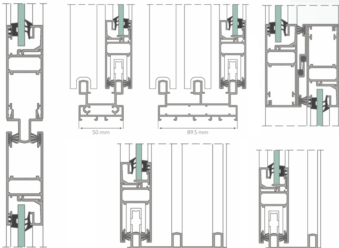
TOLÓSZÁRNYON KERESZTÜLI METSZET
