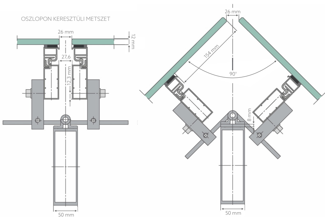
OSZLOPON KERESZTÜLI METSZET - SÁROK KAPCSOLAT
